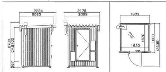
HMS-1 排気ダクトφ100
