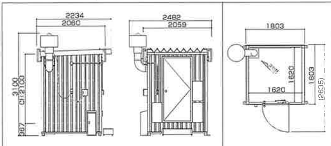
HMS-1 排気ダクトφ200 (オプションあり)
